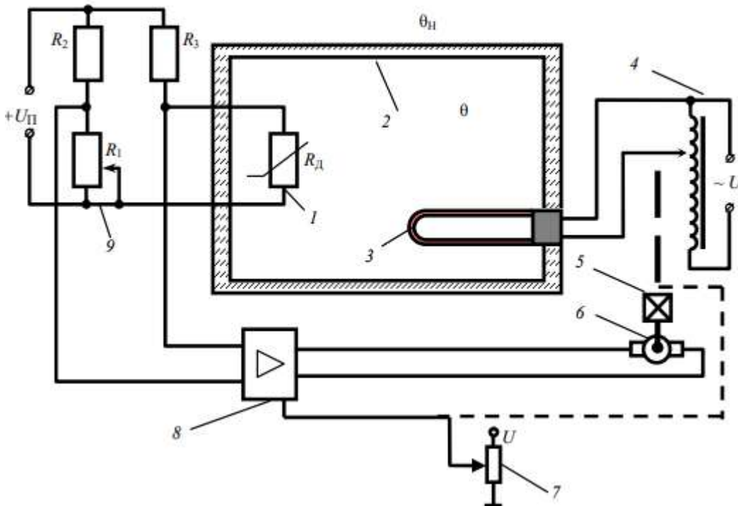
Рис. 4. Схема системы автоматического регулирования температуры в климатической камере: 1 – датчик (термометр сопротивления); 2 – климатическая камера; 3 – электрический нагреватель; 4 – автотрансформатор; 5 – редуктор; 6 – электродвигатель; 7 – потенциометр местной обратной связи; 8 – дифференциальный усилитель; 9 – мостовая измерительная схема
