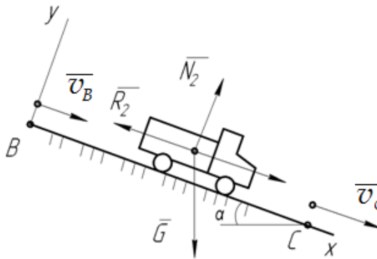
Рисунок 1.3 - Расчетная схема для участка BC
