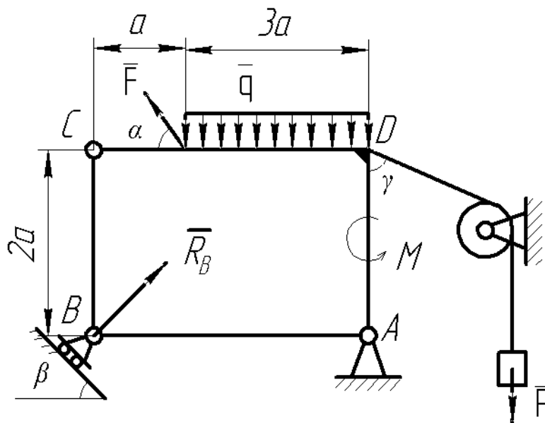
Рисунок 2.10 – Схема фермы к примеру выполнения задания 1
