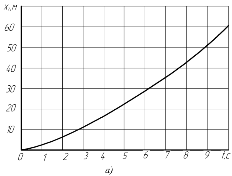
Рисунок 1.5 – Графики движения (а), скорости (б) и ускорения (в) автомобиля на участке АВ пути
