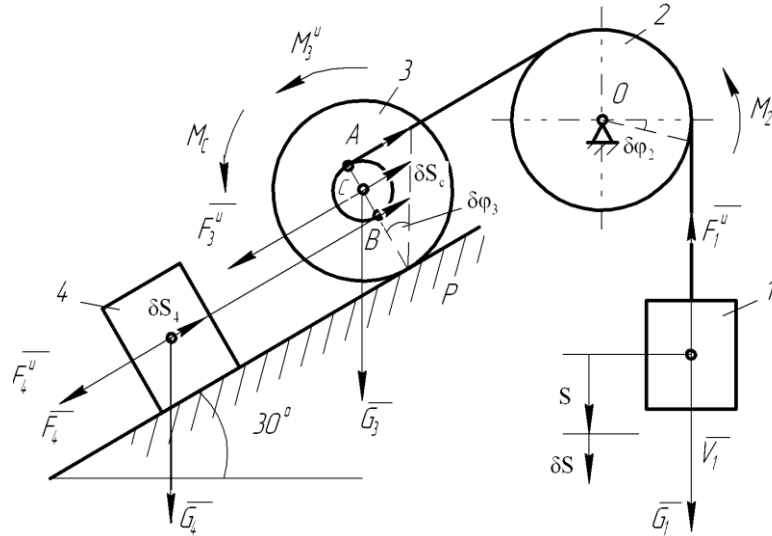
Рисунок 2.7 – Схема механической системы к выполнению п.2 задания 2
