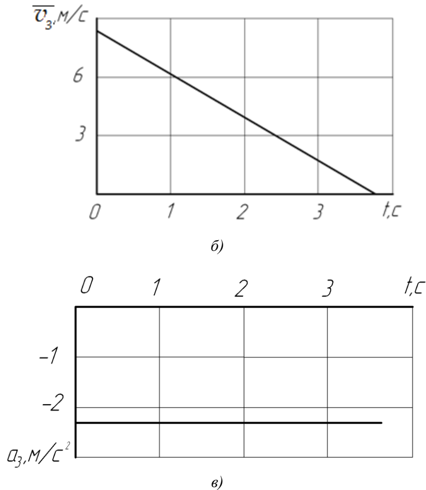
Рисунок 1.7 – Графики движения (а), скорости (б) и ускорения (в) автомобиля на участке CD пути
