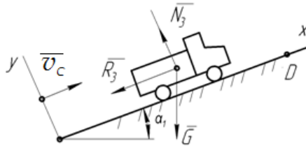
Рисунок 1.4 – Расчетная схема для участка CD
