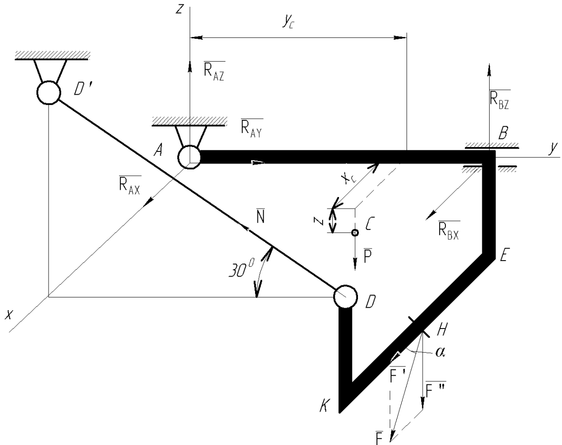
Рисунок 3.10 – Расчетная схема к заданию 2
