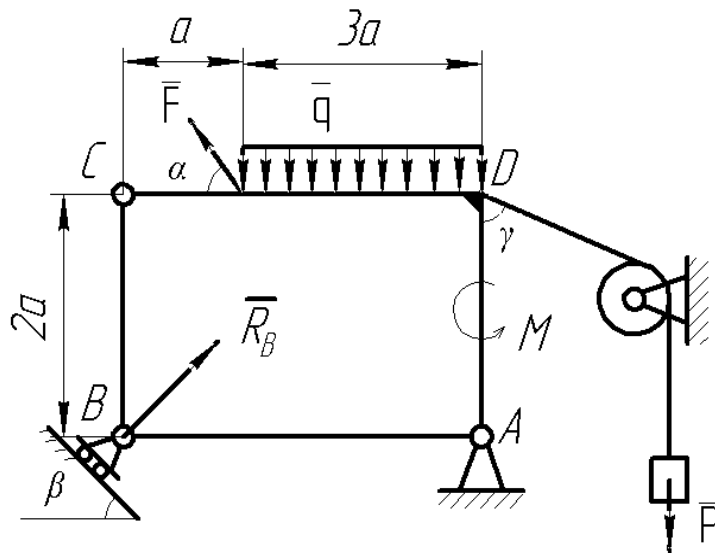
Рисунок 2.10 – Схема фермы к примеру выполнения задания 1
