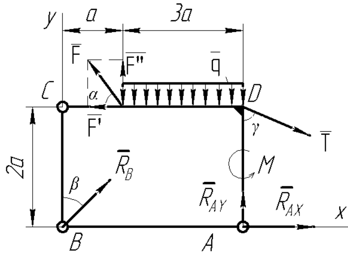
Рисунок 2.11 – Расчетная схема к примеру выполнения задания 1
