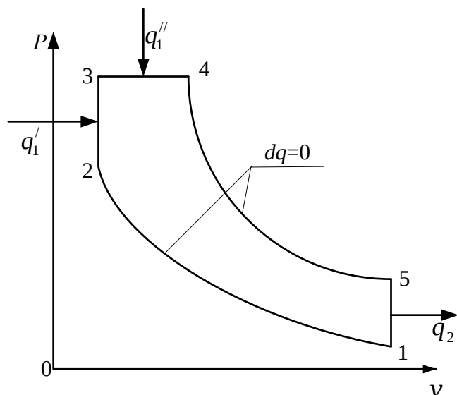
Рисунок 1 – Идеальный цикл ДВС со смешанным подводом тепла в P - v координатах.
