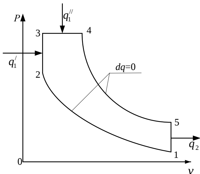
Рисунок 1 – Идеальный цикл ДВС со смешанным подводом тепла
