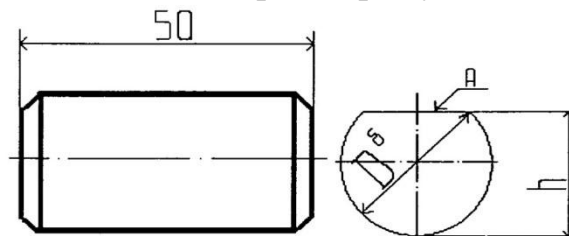
Рис.2. Эскиз детали
