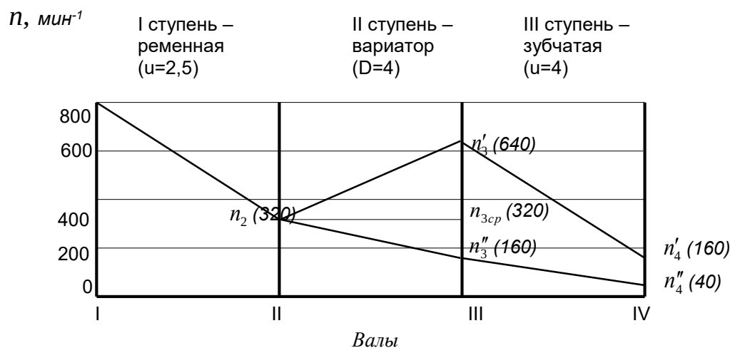
Рисунок 1 - Диаграмма частот вращения валов привода
