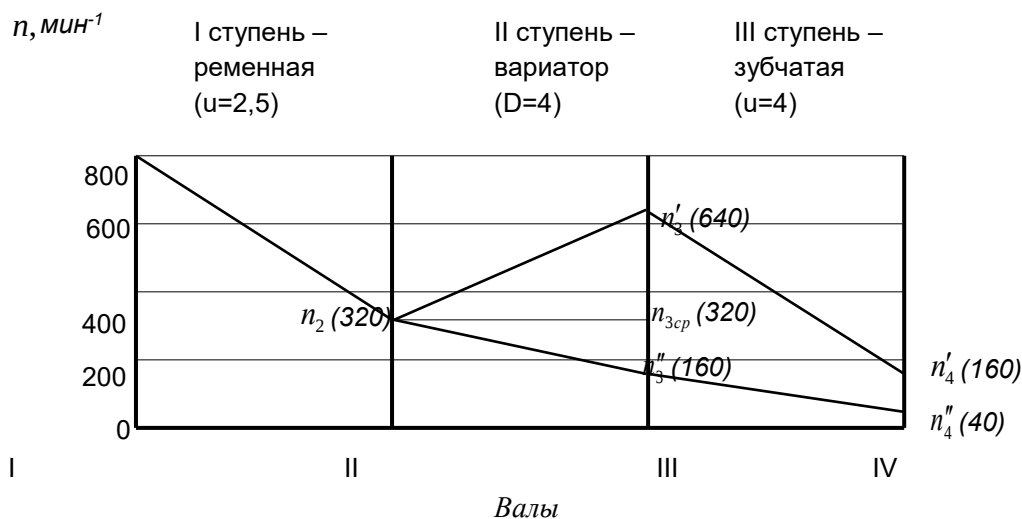
Рисунок 1 - Диаграмма частот вращения валов привода
