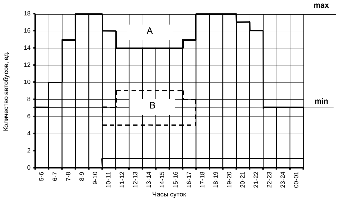
Рис. 4. Промежуточное распределение автобусов
