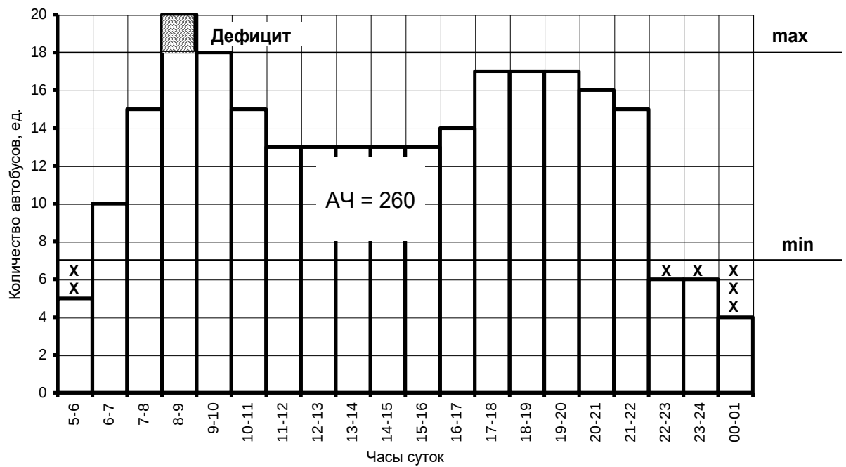
Рис. 3. Расчетное распределение автобусов по часам периода движения
