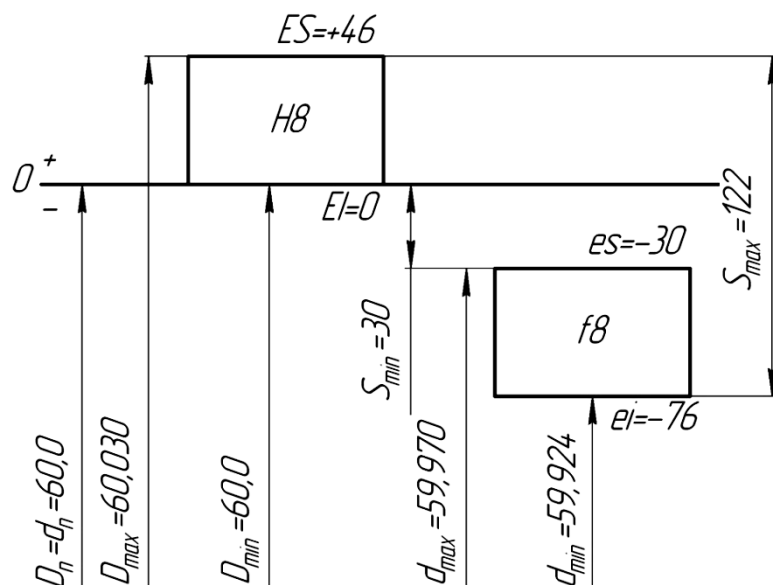
Рис.3.2 Схема полей допусков соединения
