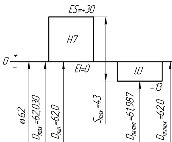
Рис. 6.2 Схема расположения полей допусков сопряжения отверстие корпуса – наружное кольцо подшипника
