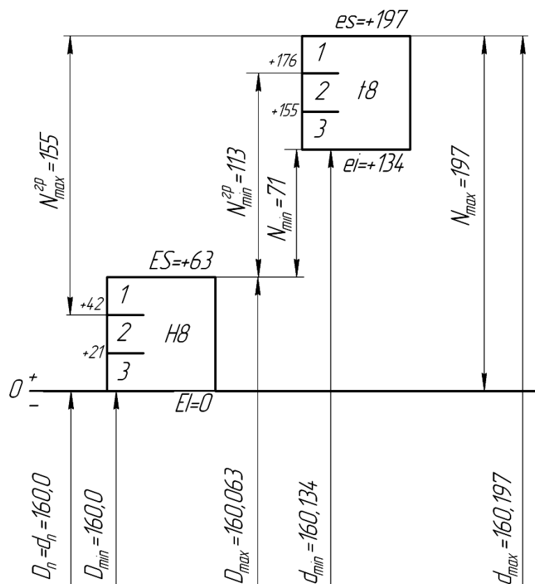
Рис. 9.1 - Схема расположения полей допусков соединения \varnothing 160 \frac{H8}{t8} при сборке методом групповой взаимозаменяемости
