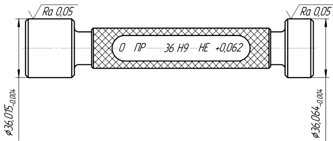
Рис. 2.4 Эскиз калибра – пробки
