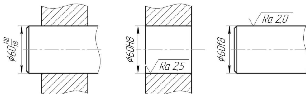
Рис.3.3. Обозначение посадки и полей допусков деталей на чертежах
