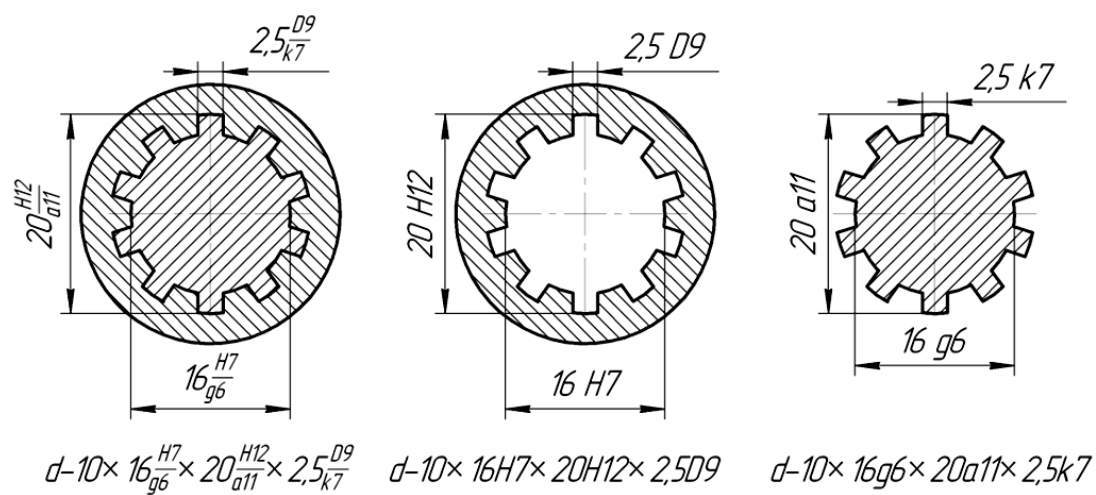
Рис. 8.4 Обозначение посадки и предельных отклонений размеров на сборочном и рабочих чертежах шлицевого соединения
