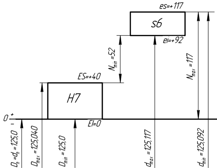
Рис. 4.2 Схема полей допусков соединения
