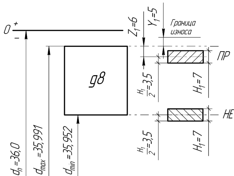
Рис.2.5 Схема расположения допусков калибров для контроля вала
