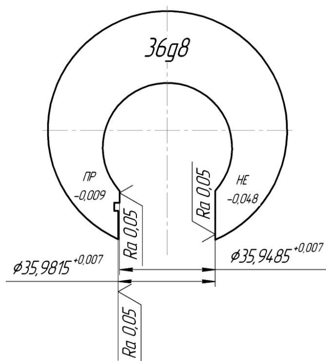
2.6. Эскиз калибра-скобы
