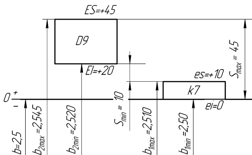
Рис. 8.3 – Схема расположения полей допусков ширины шлица
