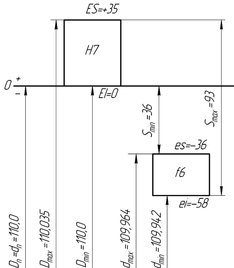
Рис. 5.1 Схема расположения полей допусков соединения
