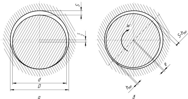
Рис.3.1 Положение вала: a – в состоянии покоя; b – в рабочем состоянии;
