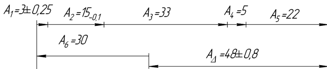
Рис. 10.1 Геометрическая схема размерной цепи
