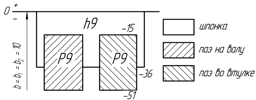
Рис. 7.1 Схема полей допусков шпоночного соединения.
