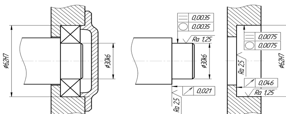
Рис.6.3 Обозначение посадки и предельных отклонений размеров на сборочном и рабочих чертежах
