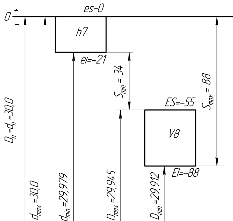
Рис. 5.2 Схема расположения полей допусков соединения
