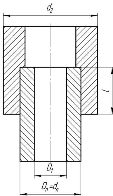
Рис. 4.1. Схема для расчета посадки с натягом
