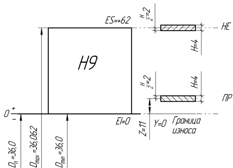
Рис. 2.3 Схема расположения полей допусков калибра для контроля отверстия
