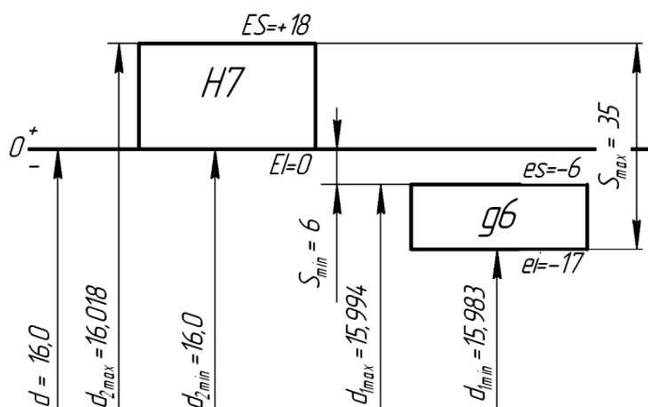
Рис. 8.1 – Схема расположения полей допусков внутреннего диаметра шлицевого соединения
