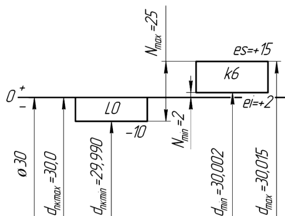
Рис. 6.1 Схема расположения полей допусков сопряжения вал - внутреннее кольцо подшипника
