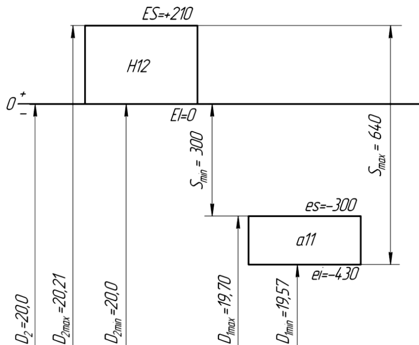
Рис. 8.2 – Схема расположения полей допусков наружного диаметра шлицевого соединения
