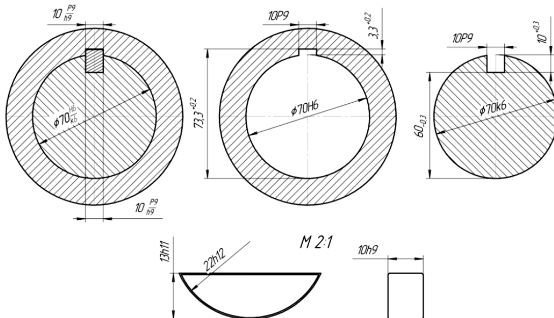
Рис. 7.2 Обозначение посадки и предельных отклонений размеров на сборочном и рабочих чертежах деталей шпоночного соединения.
