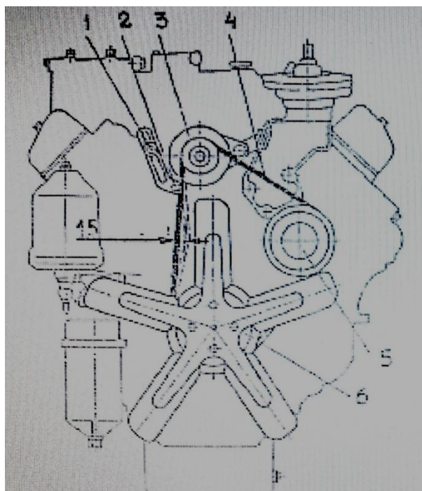
Рисунок - 18 Схема натяжения ремней привода водяного насоса и генератора:1-Болт, 2-Болт крепления бланки генератора,3-Генератор, 4-Ремни приводные, 5. Шкив водяного насоса, 6.шкиф гидромфты вентилятора.
