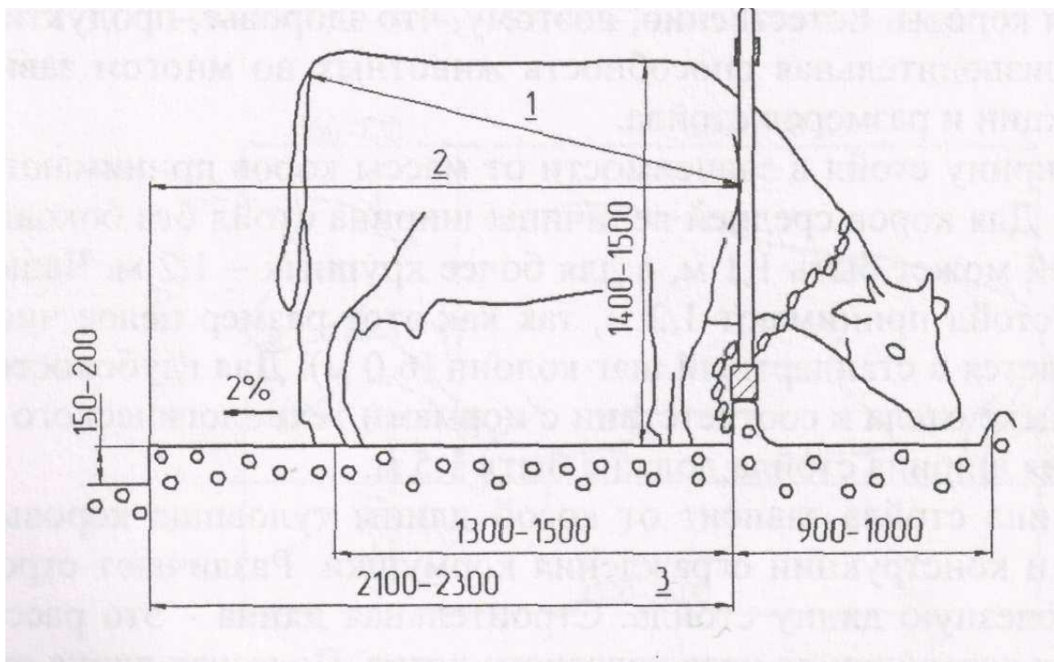
Р и с. 2. Среднее стойло с кормовой решеткой:
